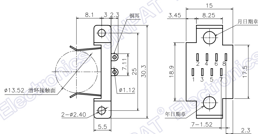
LPS-08C-S尺寸
